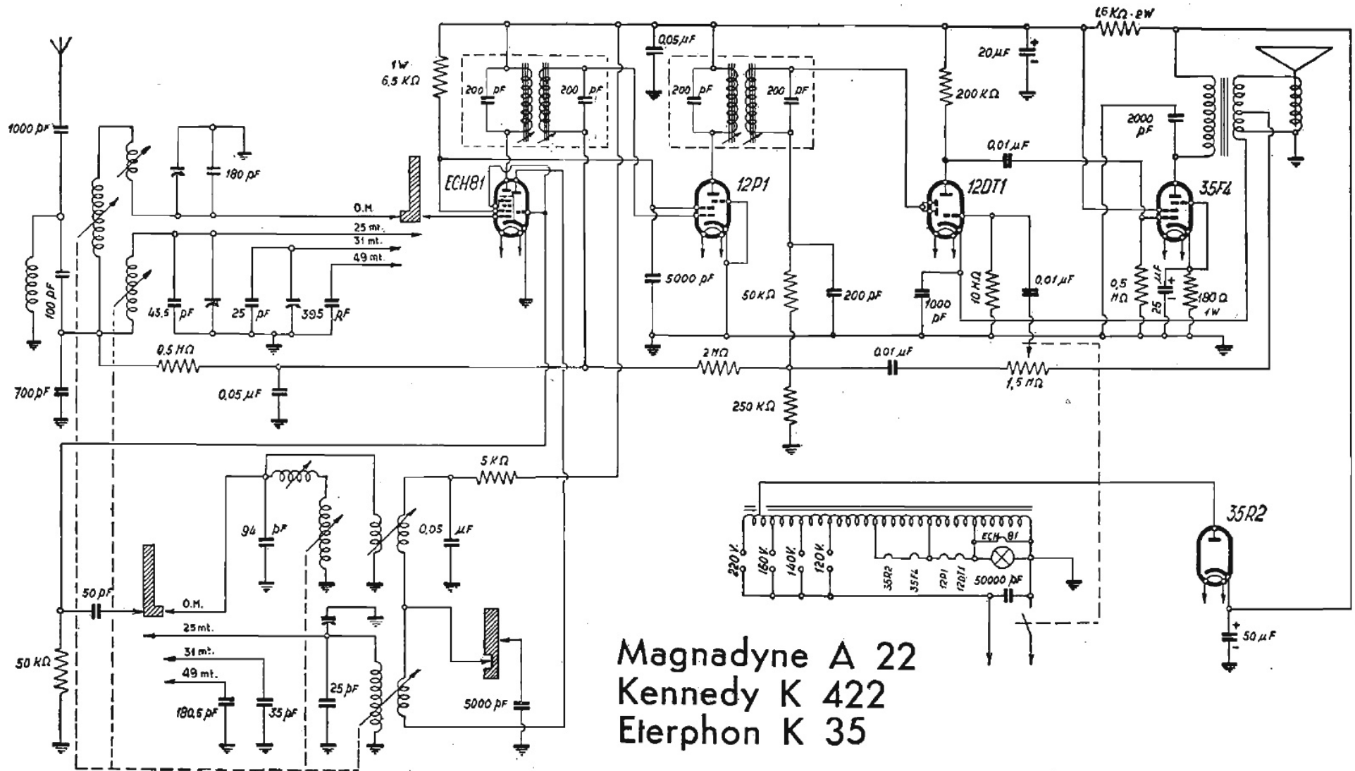
MAGNADYNE RADIO - Modd. A 22, K 35 e K 422. Ricevitore a onde medie con tre bande allargate ad onde corte. Media frequenza a 471 kc/s. Potenza d'uscita 2 watt.
